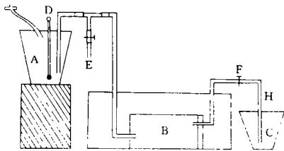
图1 流水式密闭装置
