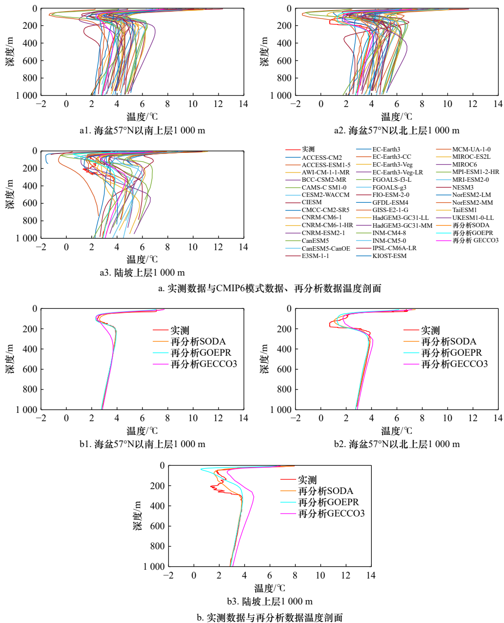
图2 2012年7月CMIP6模式数据、再分析数据与实测数据的海盆、陆坡上层1 000 m以浅温度剖面
