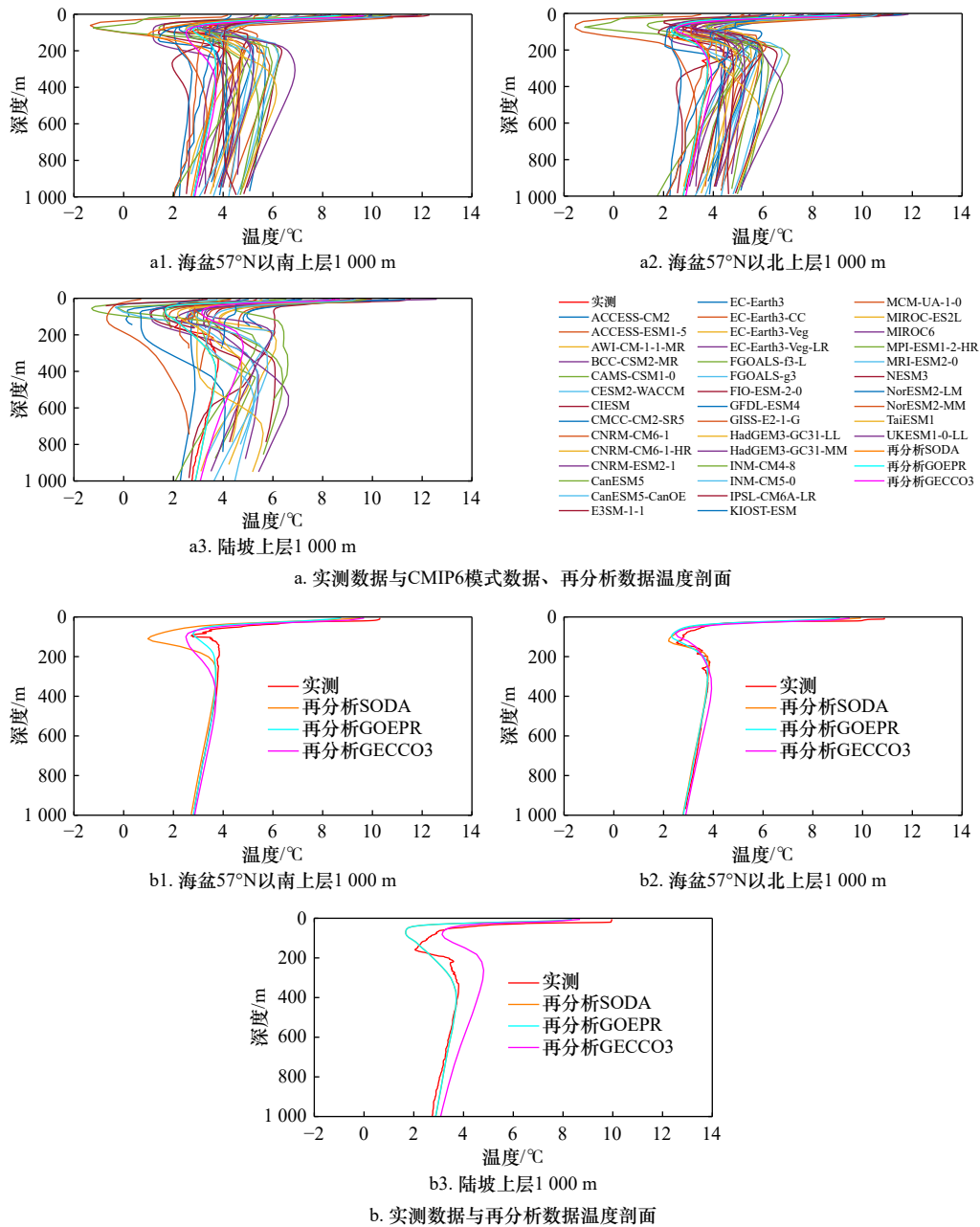
图4 2014年7月CMIP6模式数据、再分析数据与实测数据的海盆、陆坡上层1 000 m以浅温度剖面
