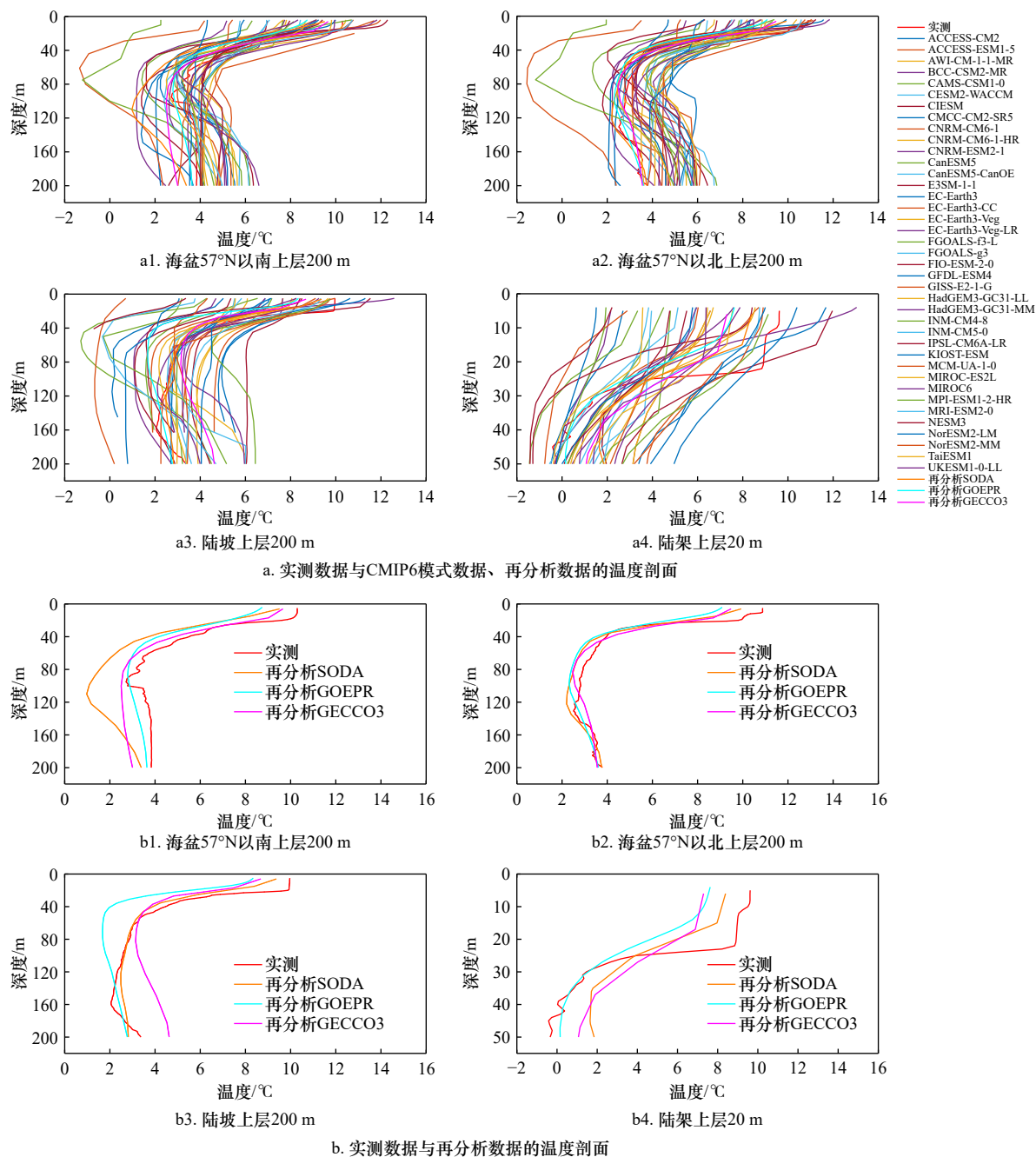
图3 2014年7月CMIP6模式数据、再分析数据与实测数据的海盆、陆坡和陆架上层200 m以浅温度剖面
