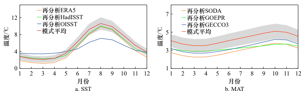
图 7 1950–2023 年白令海区域 (51°~66°N, 162°E~152°W) 基于再分析与模式平均数据 (包含模式: CIESM, CMCC-CM2-SR5, CanESM5, EC-Earth3, EC-Earth3-CC, EC-Earth3-Veg-LR, HadGEM3-GC31-MM 和 TaiESM1) 的月平均时间序列
