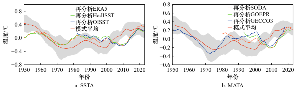
图8 1950–2023年白令海区域(51°~66°N, 162°E~152°W)基于再分析与模式平均数据(包含模式: CIESM、CMCC-CM2-SR5、CanESM5、EC-Earth3、EC-Earth3-CC、EC-Earth3-Veg-LR、HadGEM3-GC31-MM和TaiESM1)的去除线性趋势后的年平均异常时间序列
